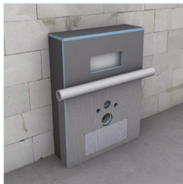
...przykleić lub przykręcić, przykleić siatkę zbrojącą...
